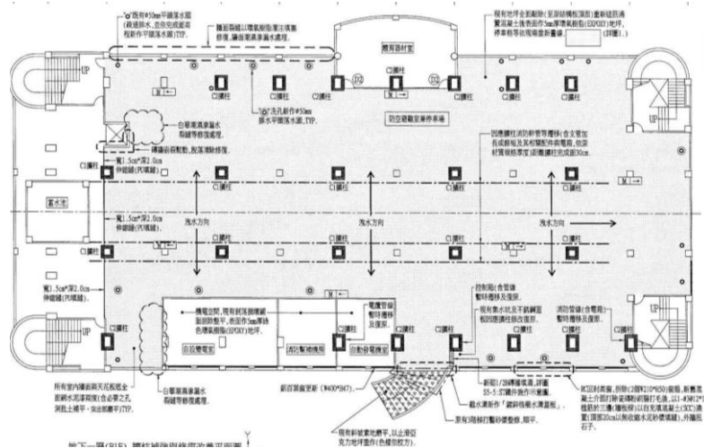
各樓層平面配置圖
