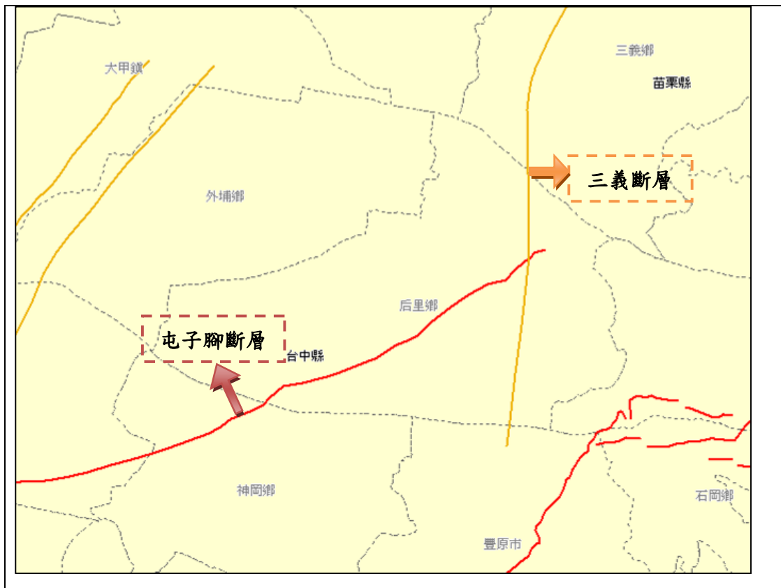
圖 2-2-1、活動斷層圖
